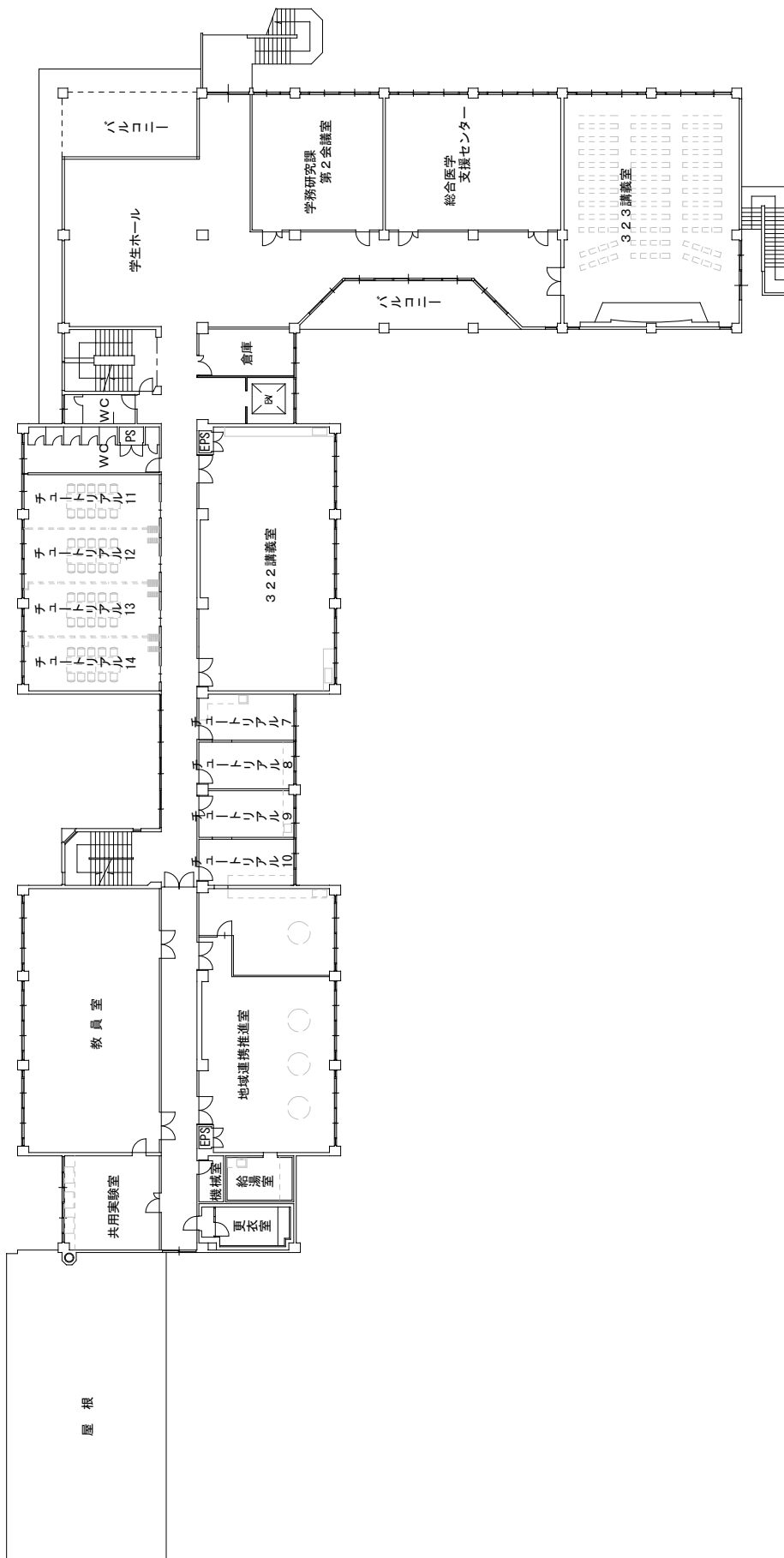
総合教育棟 2 階平面図 S=1:400
