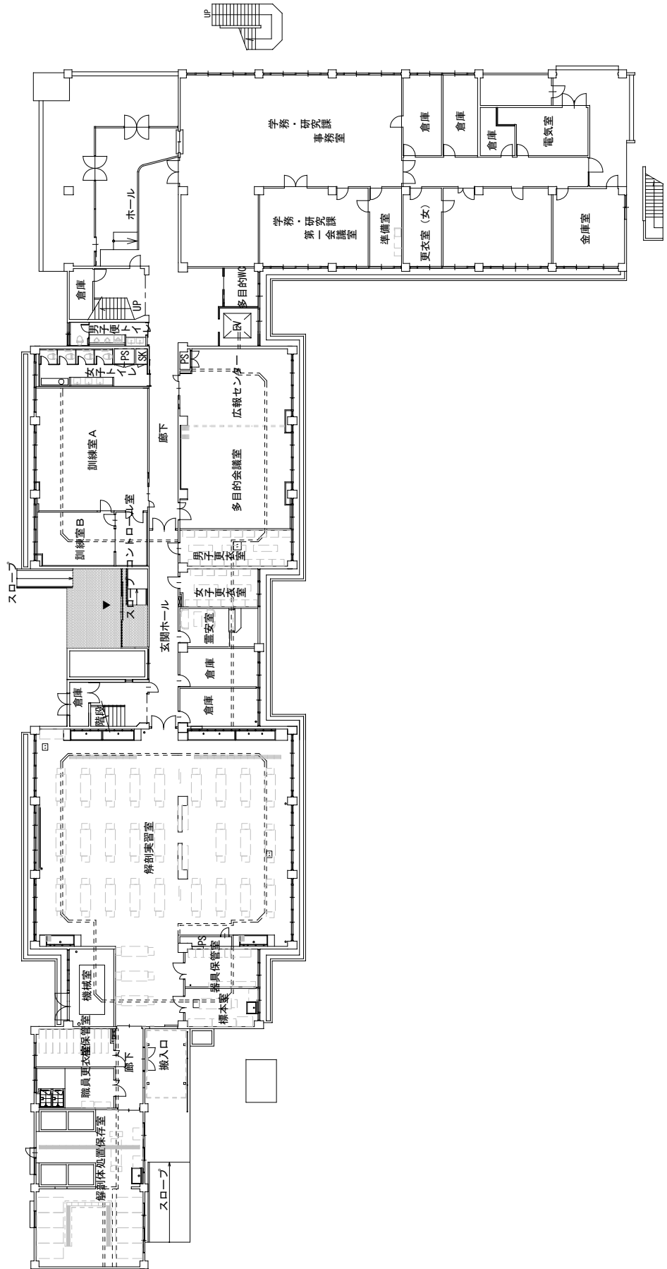
総合教育棟 1階平面図 S=1:400
